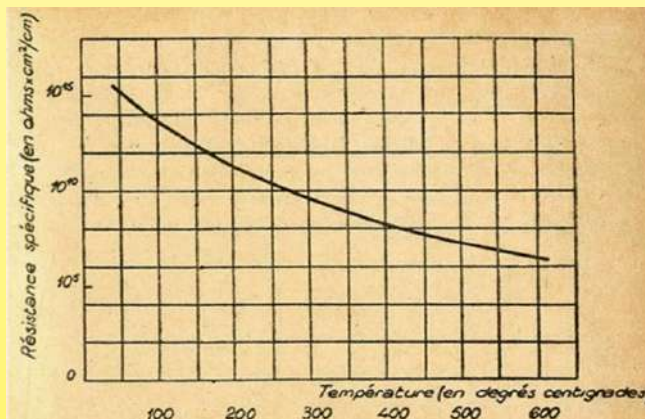
Изменение удельного сопротивления фарфора в Ом·см/см 2 в зависимости от температуры (логарифмическая кривая). В диапазоне температур между 20°C и 300°C его сопротивление делится на 10 000 (1945 г. Matériaux électrotechniques Modernes, музей Ultimheat)
