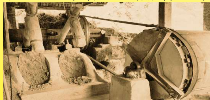
Традиционные механизмы (水碓, шуй дуй) для производства порошков, используемых для изготовления электротехнического фарфора (частная коллекция)
