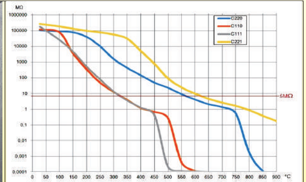
Кривые зависимости изоляционного сопротивления от температуры клеммных колодок, изготовленных из различных типов керамики (С110, С111, С220, С221), толщина 2 мм. Нормативный предел — 5 МОм.
