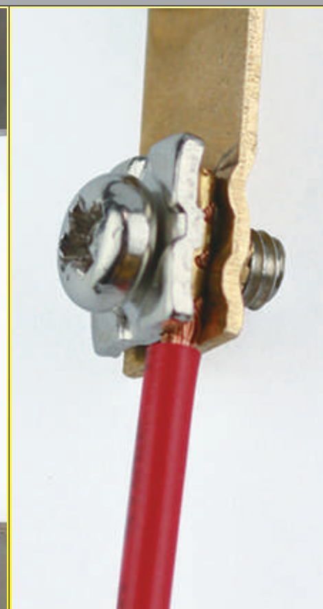
Детализированное изображение клеммного зажима
